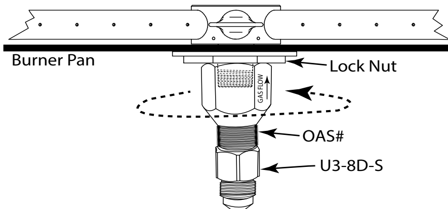
Fig. 4 Installing orifice (OAS).
